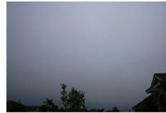
Nimbostratus
